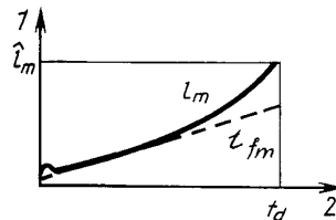
Нелинейность намагничивающего тока
