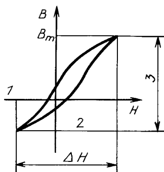
Импульсное возбуждение с постоянным подмагничивающим полем
