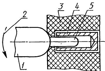
Испытательный штырь, вставленный в гнездовой контакт
