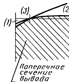
Пример правильного расположения ребра
