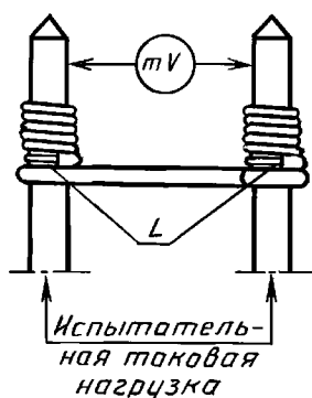
Модифицированные соединения накруткой
