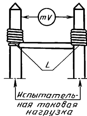
Обычные соединения накруткой
