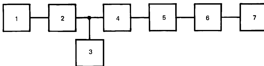
1 — измерительный компакт-диск (п. 2.2.14); 2 — измеряемый проигрыватель; 3 — эквивалент резистивно-емкостной нагрузки (п. 2.2.15); 4 — измерительный усилитель (п. 2.2.7); 5 — фильтр нижних частот (п. 2.2.11); 6 — взвешивающий фильтр (п. 2.2.12); 7 — вольтметр В2 (п. 2.2.4)
