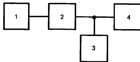
1 — измерительный компакт-диск (п. 2.2.14); 2 — измеряемый проигрыватель; 3 — эквивалент резистивно-емкостной нагрузки (п. 2.2.15); 4 — регистрирующее устройство (п. 2.2.2)
