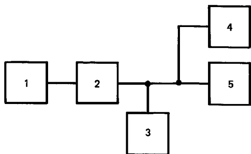
1 — измерительный компакт-диск (п. 2.2.14); 2 — измеряемый проигрыватель; 3 — эквивалент резистивно-емкостной нагрузки (п. 2.2.15); 4 — вольтметр В1 (п. 2.2.3); 5 — вольтметр В2 (п. 2.2.4)
