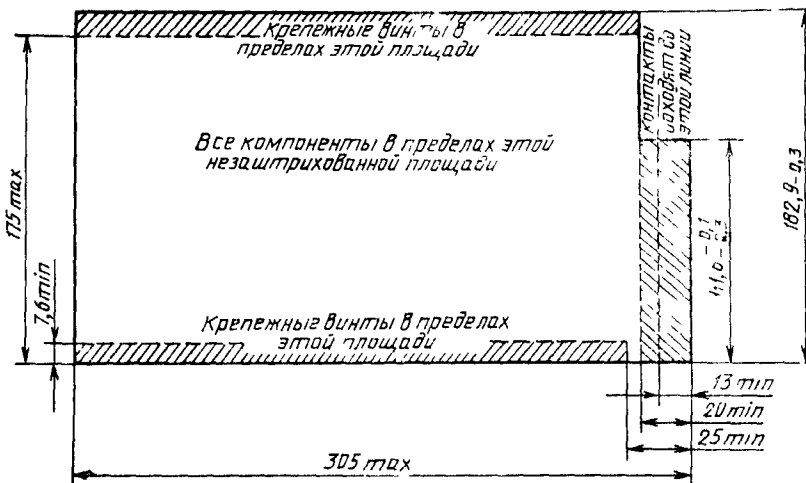
Рисунок 8 — Типовая печатная плата
