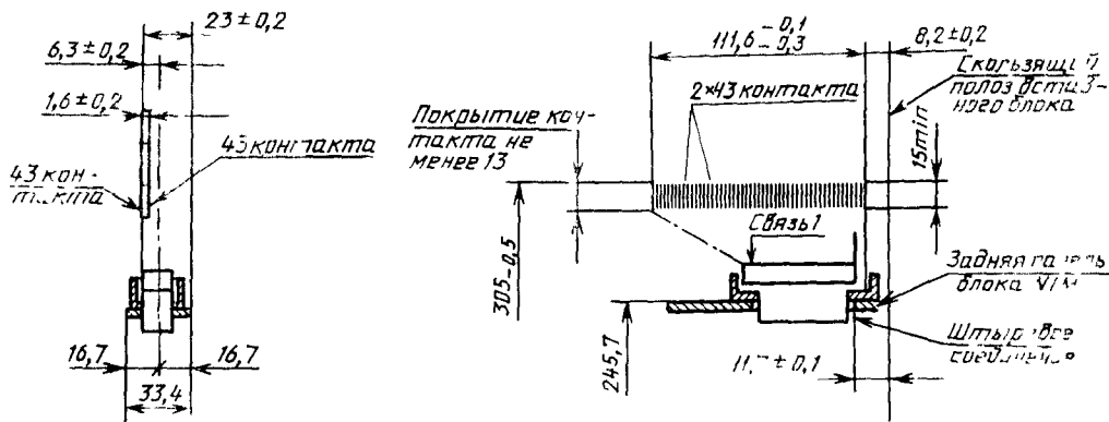
Рисунок 6 — Вентилируемый крейт. Вид спереди
