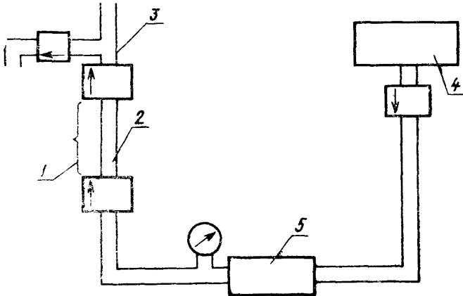
1—расстояние, регулируемое в зависимости от длины образца; 2—испытываемый образец; 3—бюретка; 4—сосуд с жидкостью; 5—насос
