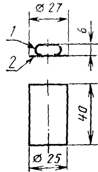
1—поворотная ручка; 2— рышля Черт. 2
