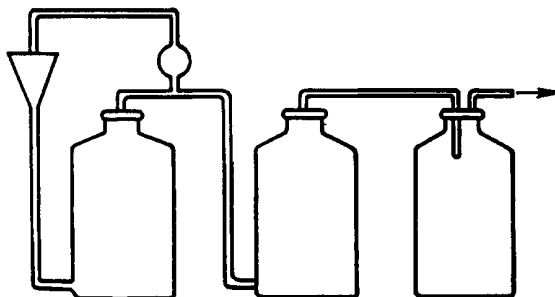
Установка для удаления ртути из сточных растворов
