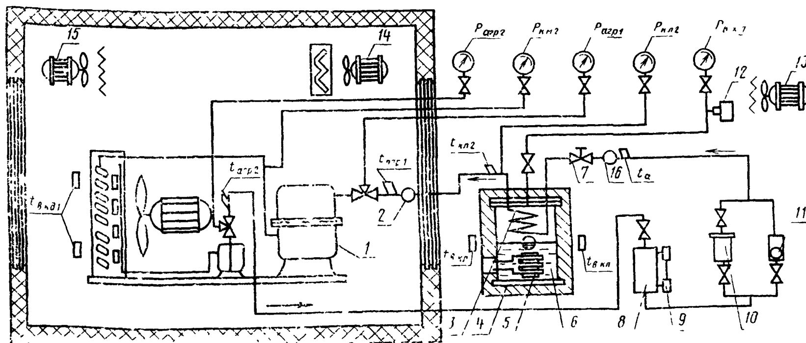
Схема стенда с электрическим калориметром
