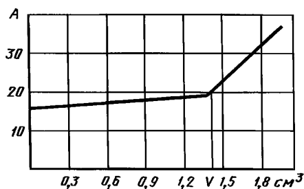
График титрования
