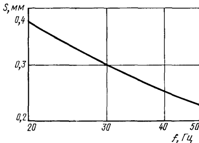
Зависимость амплитуды вибрации ( S ) от частоты ( f )
