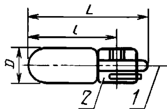
1 — базовая ось; 2 — цоколь
