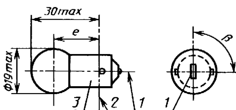
1 — базовая ось; 2 — базовая плоскость; 3 — цоколь
