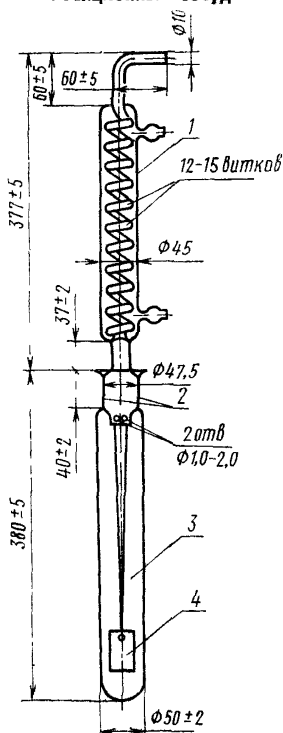
Реакционный сосуд
