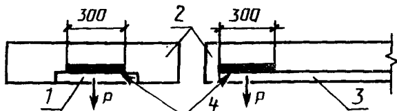
1 — короткий брусок; 2 — цапга; 3 — сквозной брусок; 4 — опорная поверхность детали (черт. 3) Черт. 4
