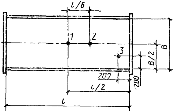
1, 2 — точки приложения нагрузки Черт. 6
