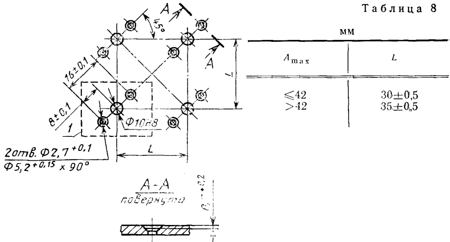
Разметка для крепления переключателей
