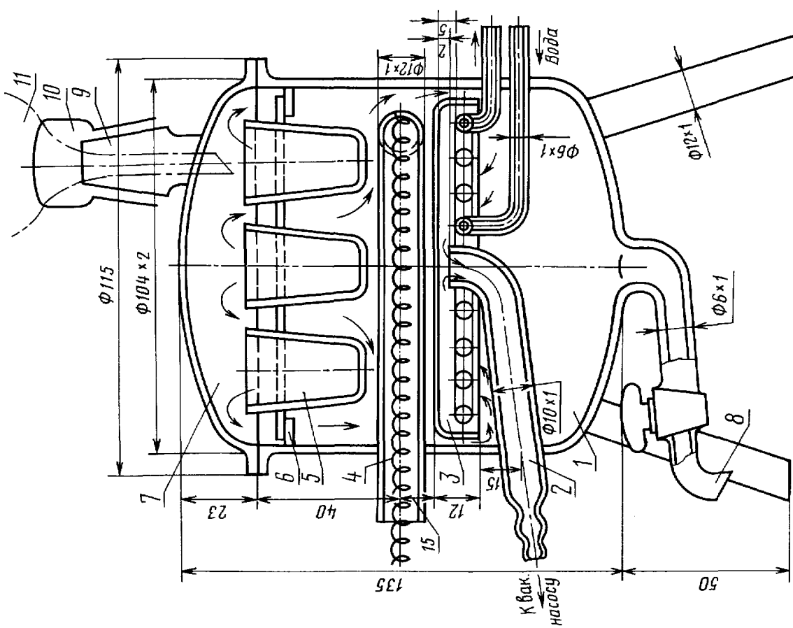
Аппарат для концентрирования примесей
