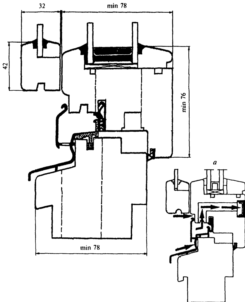
a — вариант установки климатического клапана
