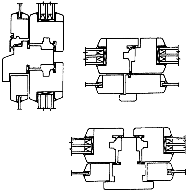
Рисунок 4 — Примеры конструктивных решений impostных и безimpostных притворов оконных блоков спаренной конструкции (вариант поворотно-откидного открывания)
