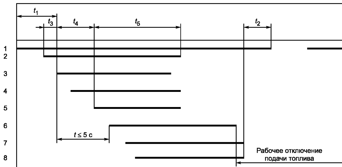
Диаграмма нормальной работы горелки
