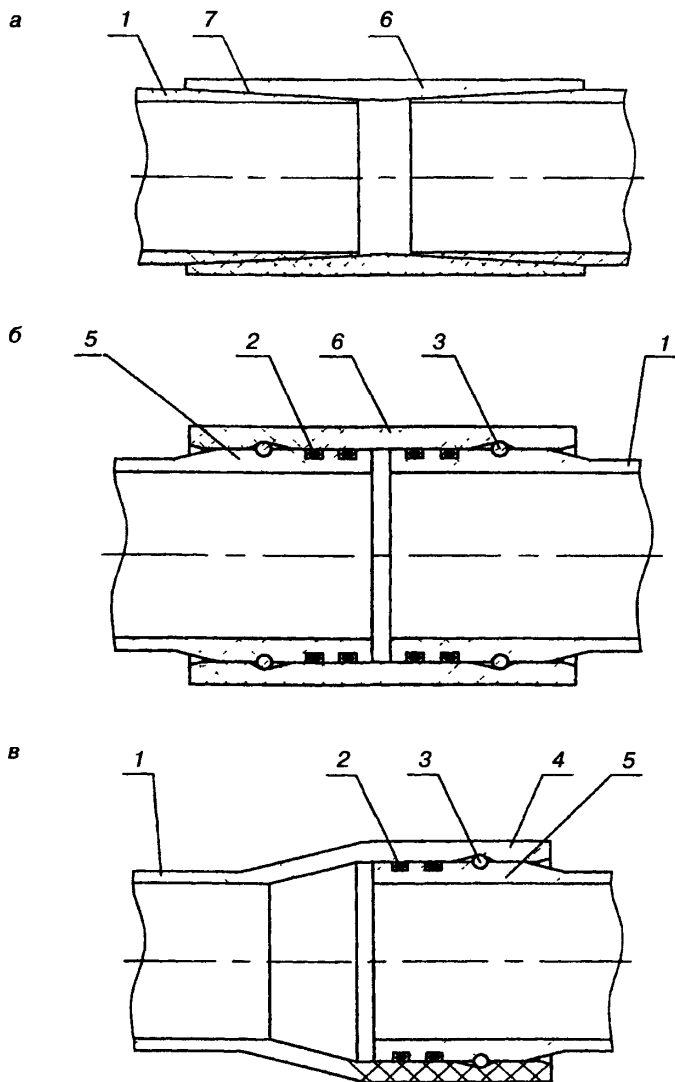
а — муфтовое клеевое; б — муфтовое; в — раструбное; 1 — труба, 2 — резиновый уплотнитель; 3 — стопорный элемент; 4 — раструб, 5 — ниппель; 6 — муфта; 7 — клеевой шов
