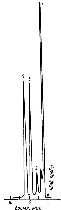
Хроматограмма фенолоанилинофор- мальдегидных смол
