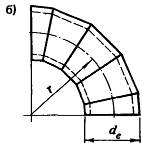
Черт. 4. Отводы
