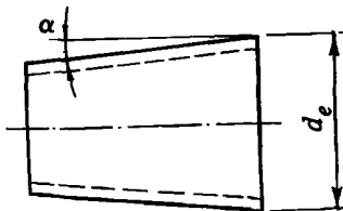
Черт. 2. Концентрический переход
