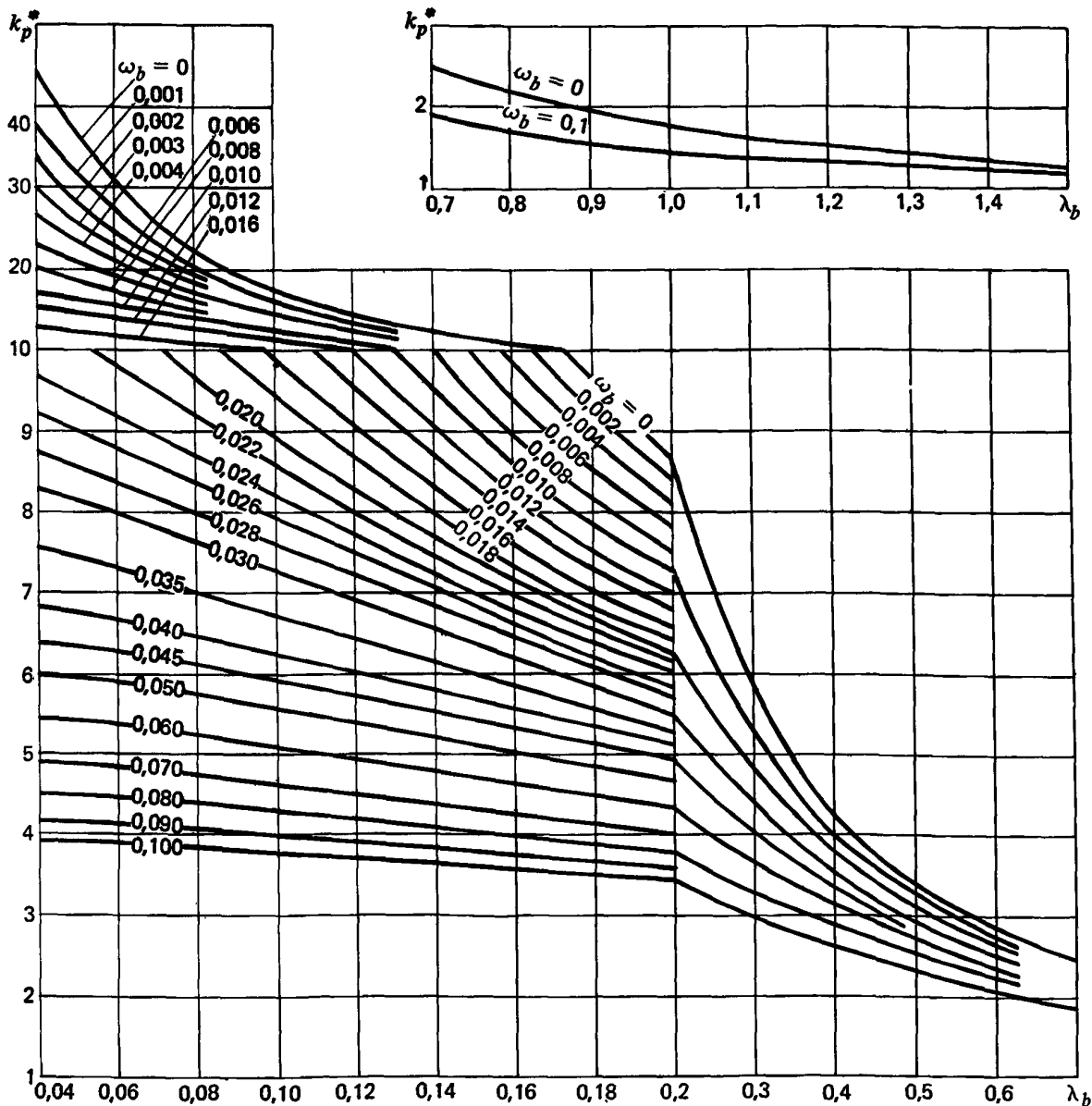
Черт. 1. График для определения значений коэффициента k_p^*
