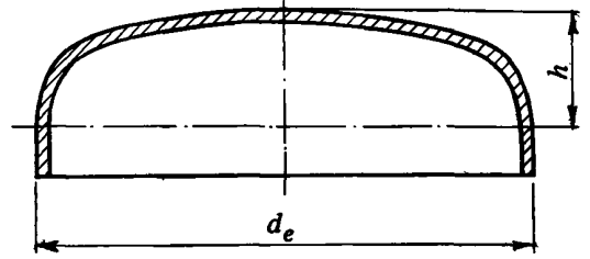
Черт. 3. Заглушка эллиптическая
