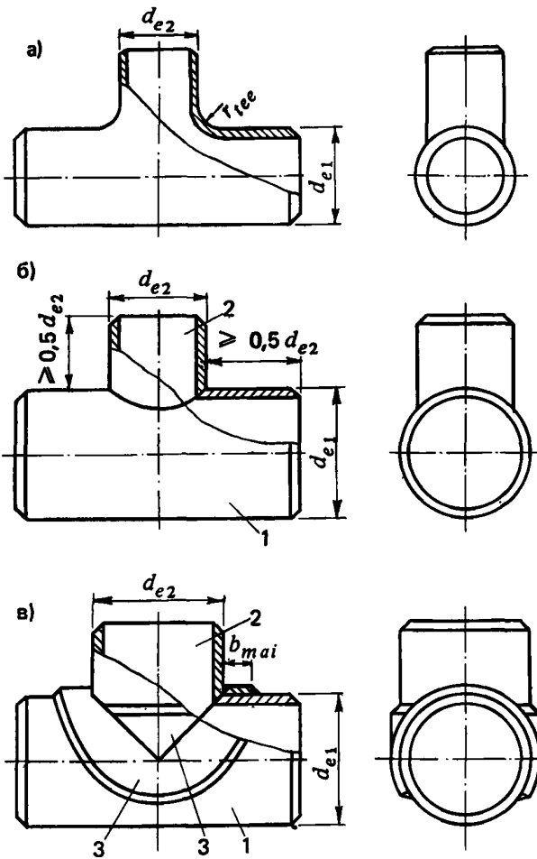
Черт. 1. Тройники
