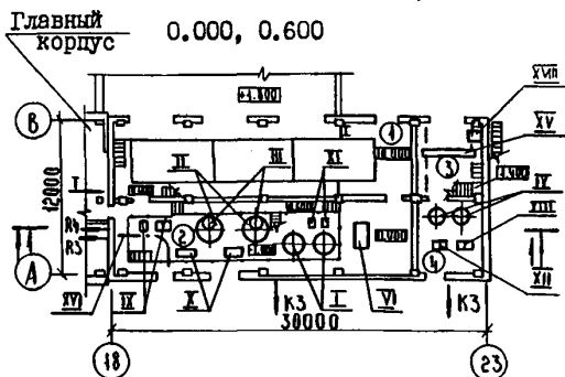
ЭКСПЛИКАЦИЯ ПОМЕЩЕНИЙ
