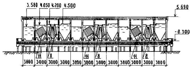
РАЗРЕЗ I-I
