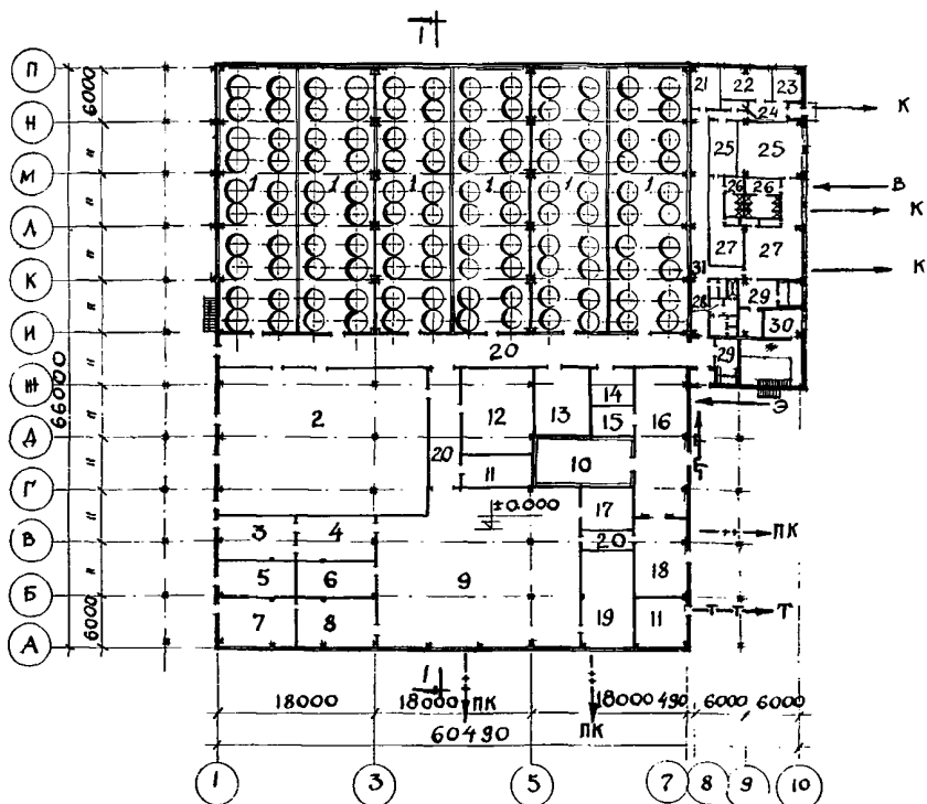
ПЛАН НА ОТМЕТКЕ \pm 0.000
