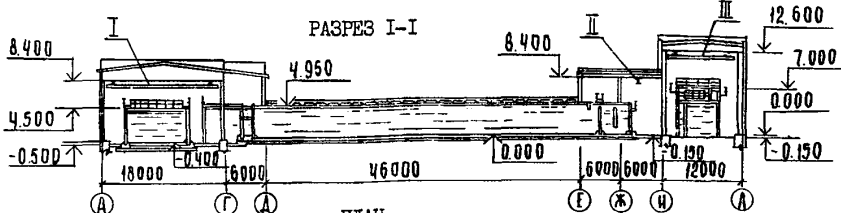
ПЛАН
