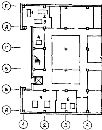
ФРАГМЕНТ ПЛАНА III ЭТАЖА НА ОТМ. 8.400
