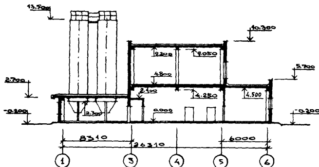
РАЗРЕЗ I-I
