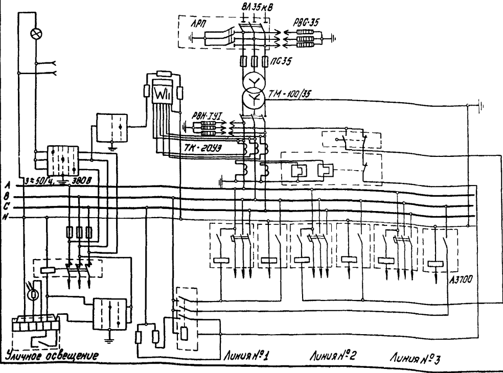
Схема электрическая принципиальная
