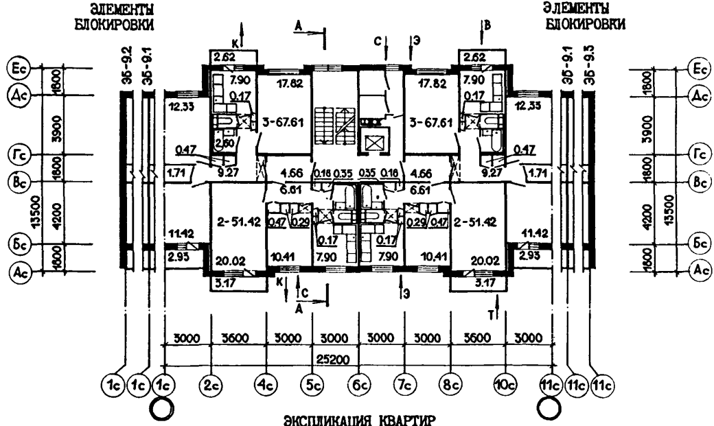
ПЛАН ТИПОВОГО ЭТАЖА неизменяемая часть
