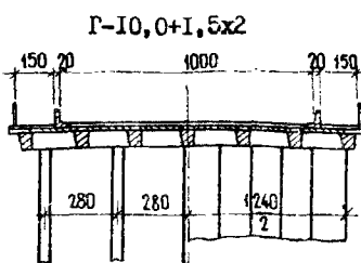
ПОПЕРЕЧНЫЕ РАЗРЕЗЫ
